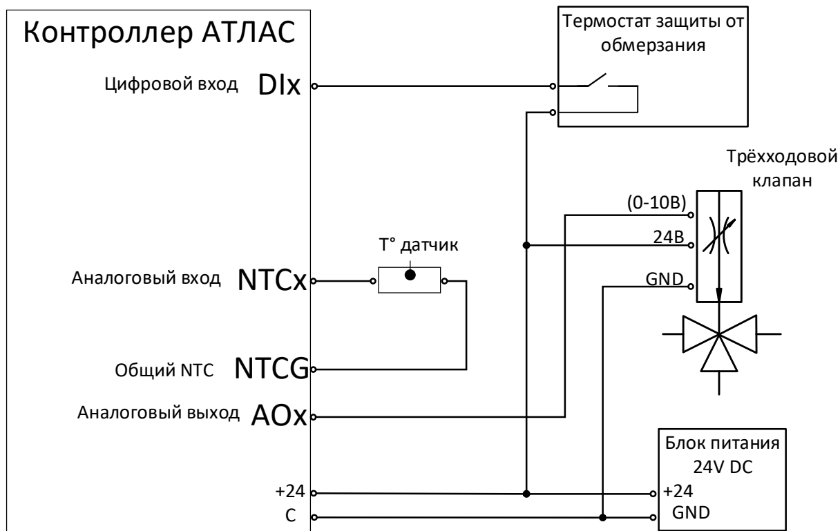
Рисунок 3.2 - Схема подключения клапана, T° датчика и термостата к контроллеру
